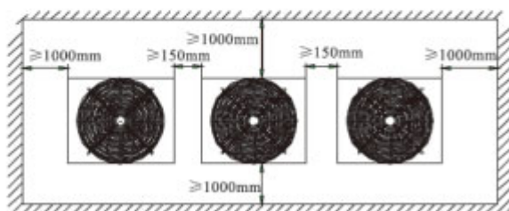
Przestrzeń serwisowa dla agregatów zestawianych w moduły
