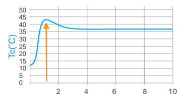
Dla modułu zewn. 134 kW, 100% wydajności osiągnięte jest w ok. 70s.
