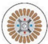
Scentralizowane uzwojenie DC
