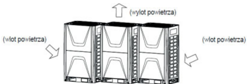
Schemat przepływu powietrza: wlot powietrza z boku i z tyłu, wylot gorą agregatu
