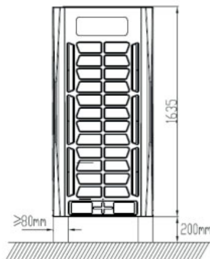
Sposób podparcia agregatu
